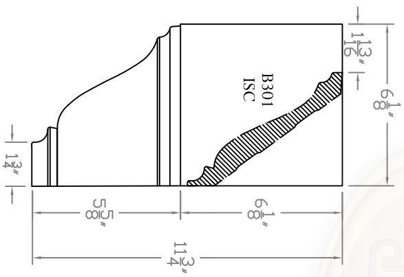
SIDE VIEW ISC Scale: 1:4
