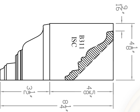
SIDE VIEW ISC
