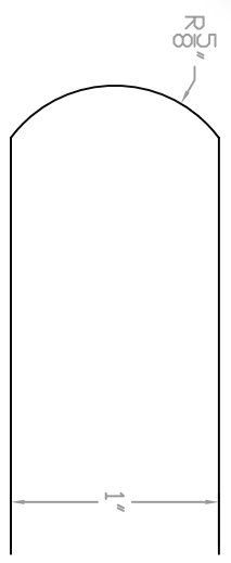
A BULLNOSE DETAIL Scale: 1:1
