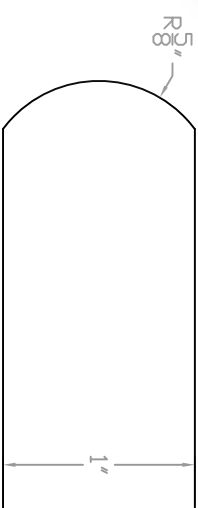
A BULLNOSE DETAIL Scale: 1:1
